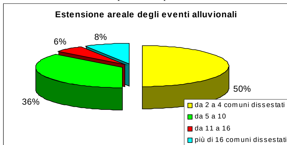
Figura 6.19 - Estensione areale degli effetti degli eventi alluvionali
